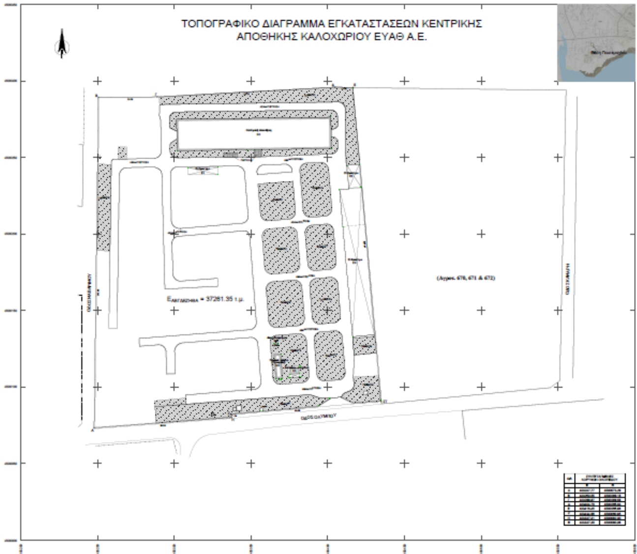
Τοπογραφικό διάγραμμα εγκαταστάσεων Κεντρικής Αποθήκης Καλοχωρίου
