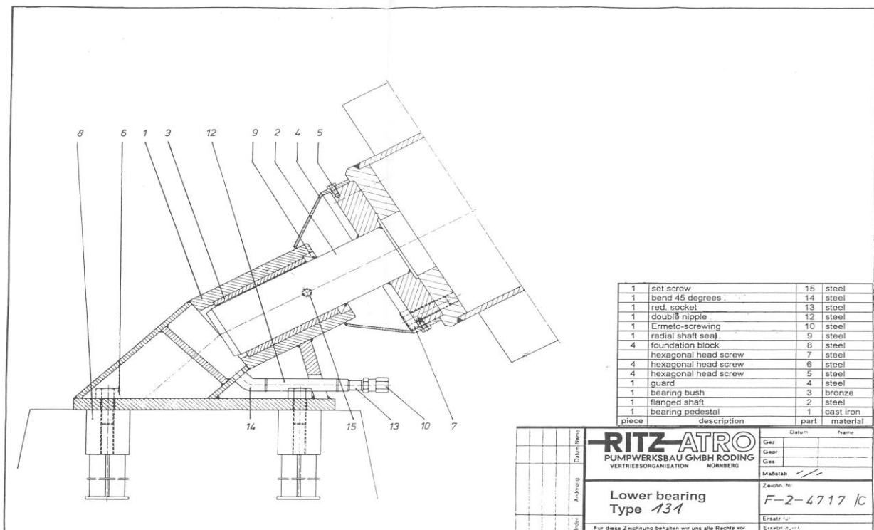
Εικόνα 3: Σχέδιο Κάτω εδράνου κοχλίου ενδιάμεσης ανύψωσης
